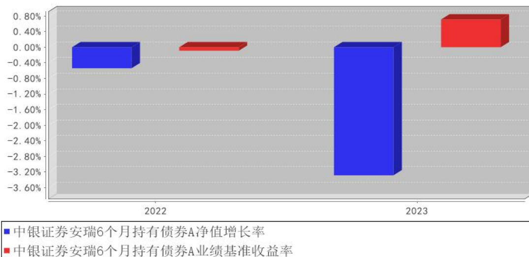
中银证券安瑞6个月持有债券A基金每年净值增长率与同期业绩比较基准收益率的对比图
