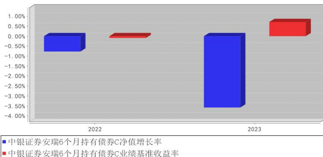
中银证券安瑞6个月持有债券C基金每年净值增长率与同期业绩比较基准收益率的对比图
