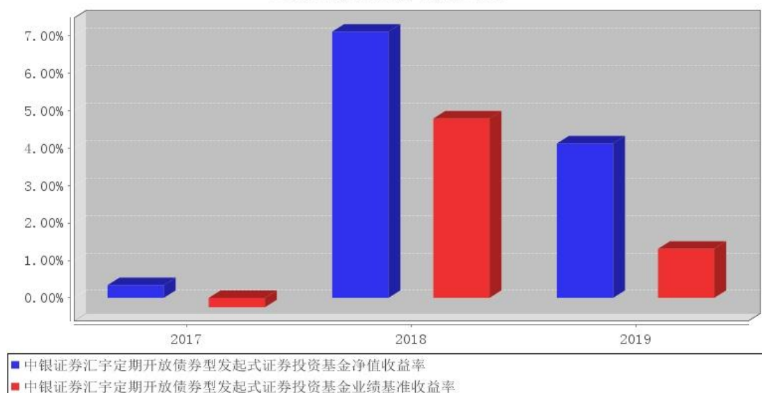
中银证券汇宇定期开放债券型发起式证券投资基金基金每年净值增长率与同期业绩比较基准收益率的对比图
